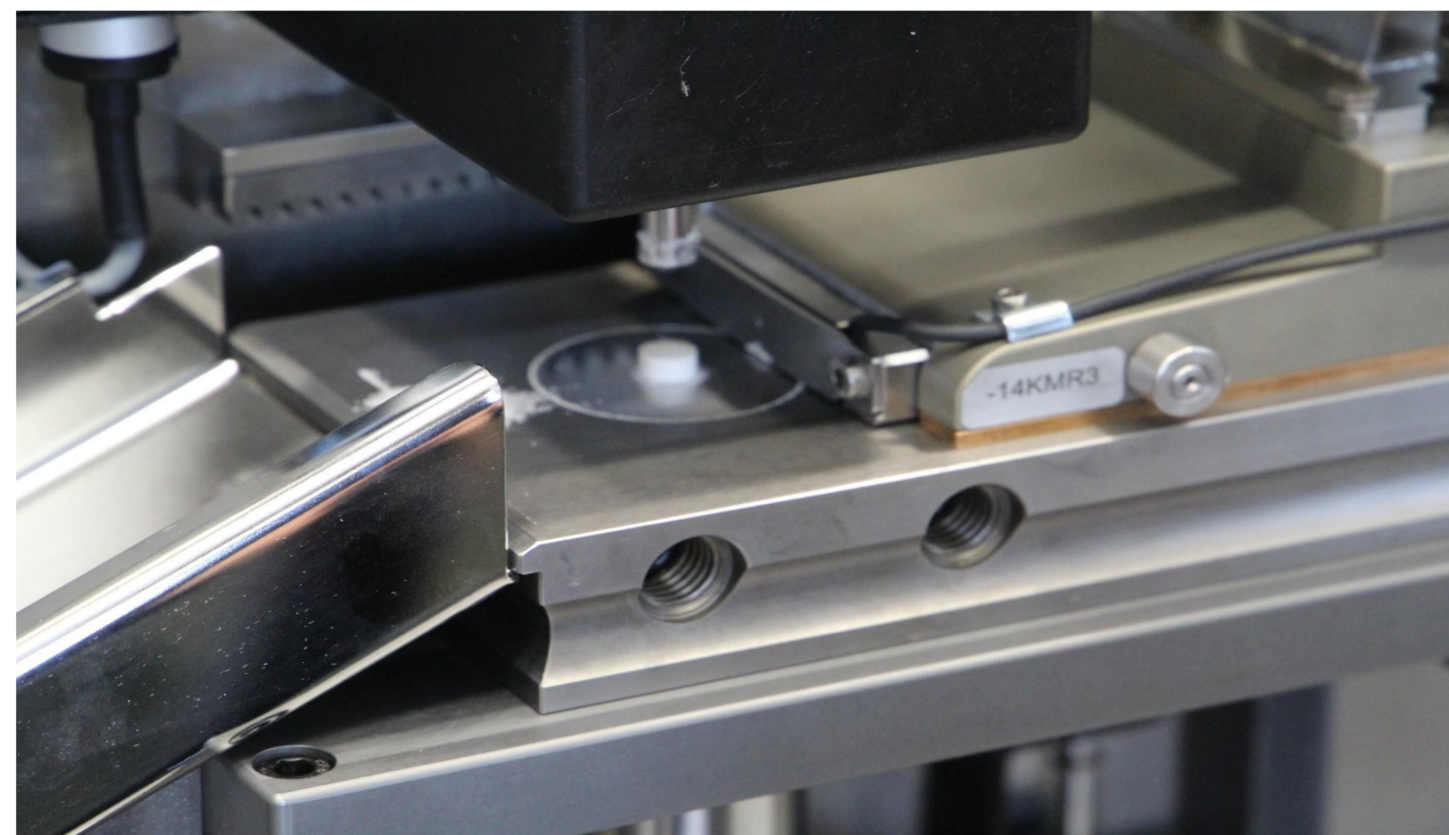
Verpresste Tablette auf Matritzentisch vor dem Auswurf
