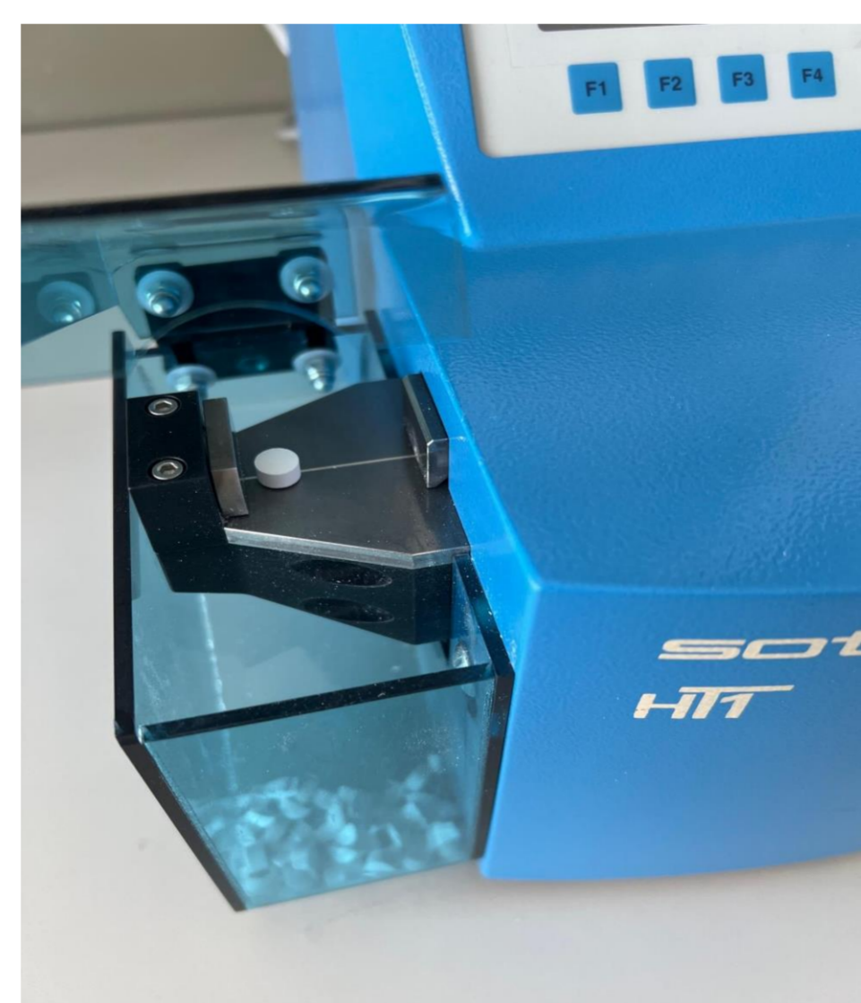
Sotax HT1 Bruchfestigkeitstester
