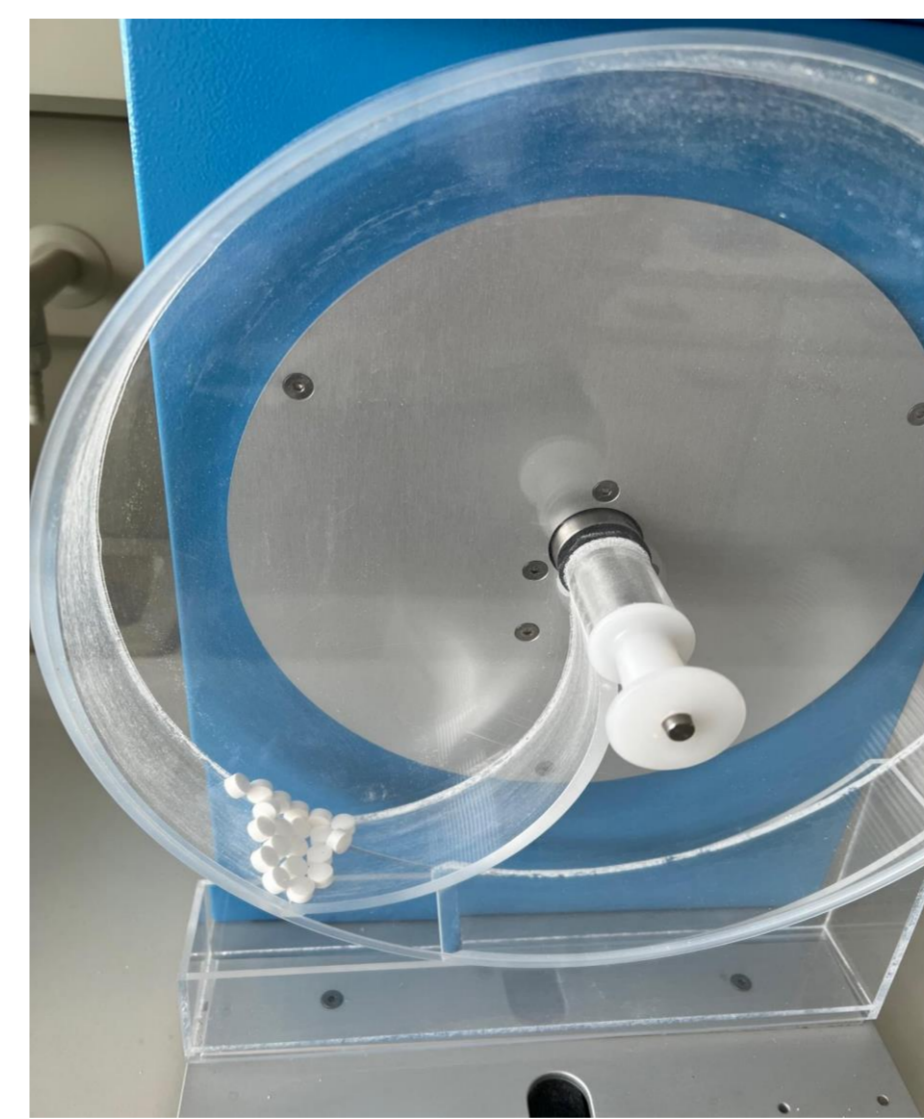
Sotax FT2 Abriebtester
